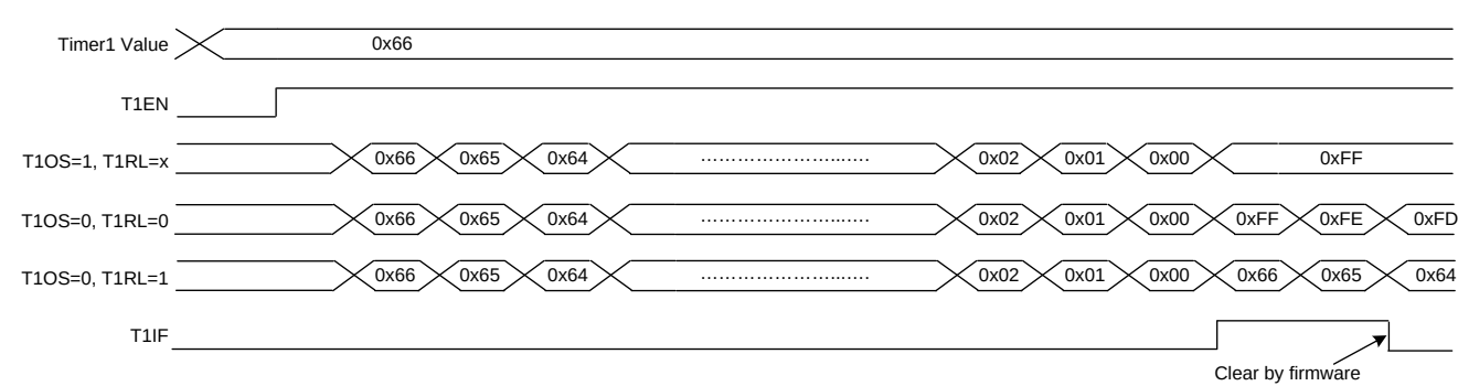
图 12 定时器 1 时序图
