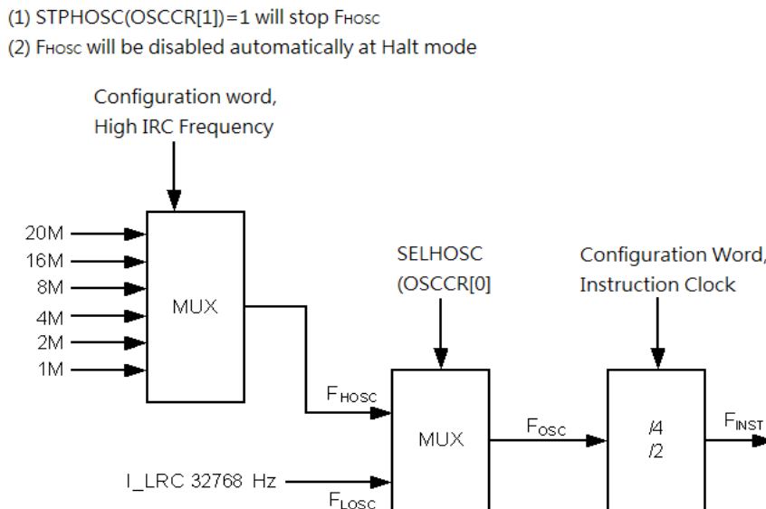
图 16 TX-P01I83 振荡配置结构图
