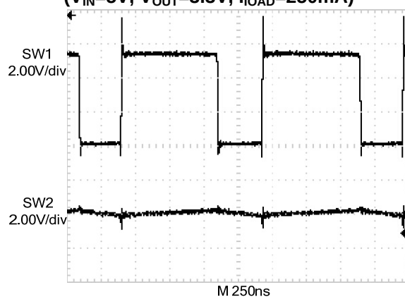
降压模式下的开关引脚
