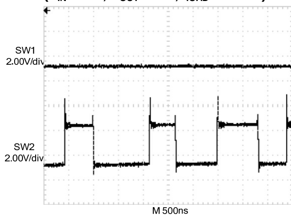
升压模式下的开关引脚
