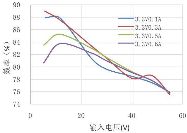
输入电压VS效率
