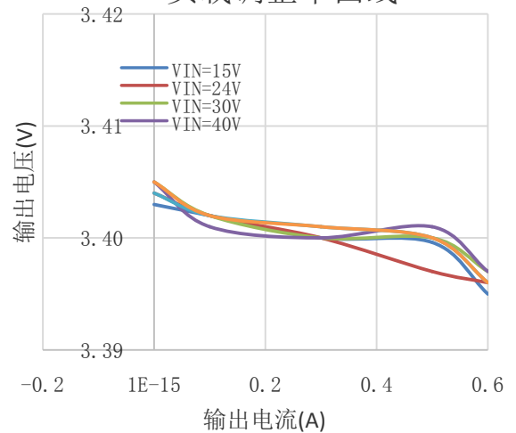
负载调整率曲线
