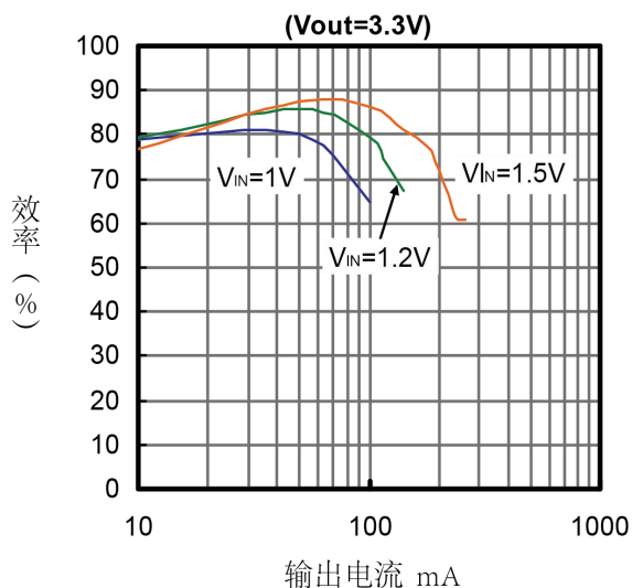
效率与输出电流曲线图
