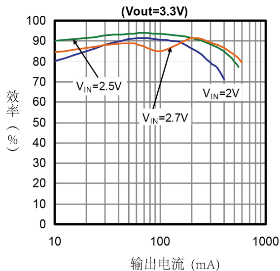
效率与输出电流曲线图
