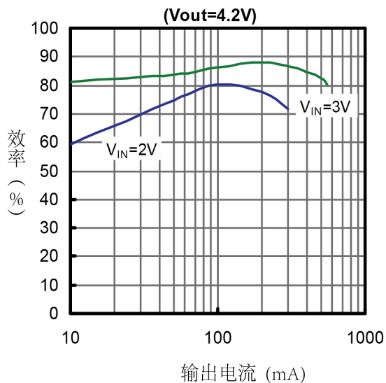
效率与输出电流曲线图
