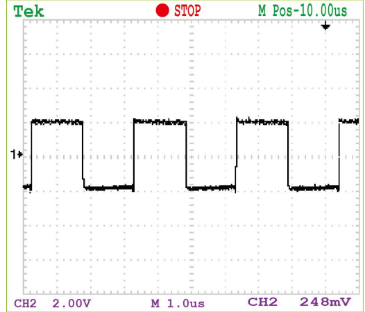
开关噪声 (VIN=4.2V,ILOAD=100mA)
